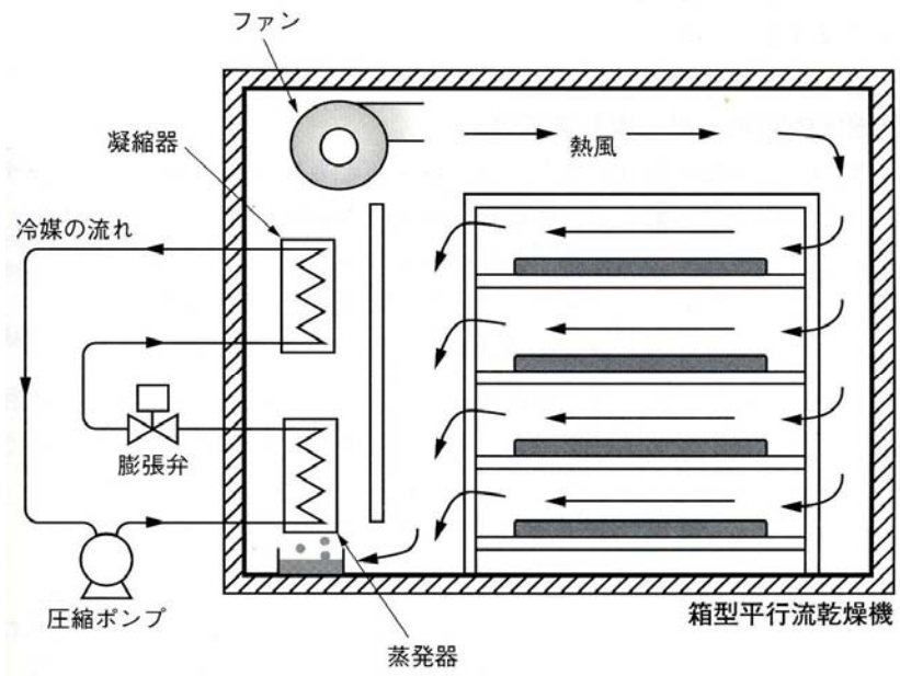
図 6.6 ヒートポンプを利用した乾燥機
